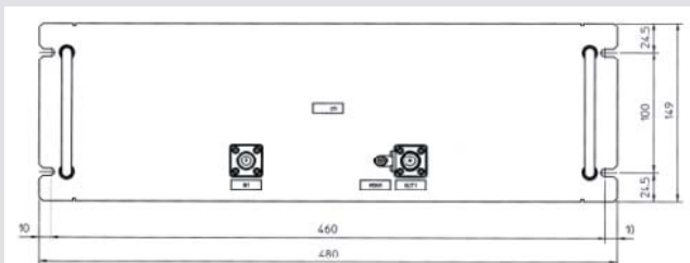
外観図 (前面)
