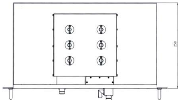
外観図 (上面)
